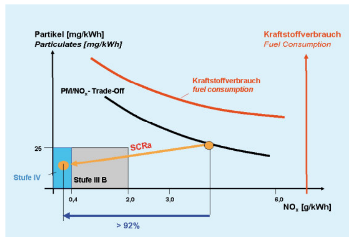
SCRa: 2-Stufen Hochleistungs-SCR-System
