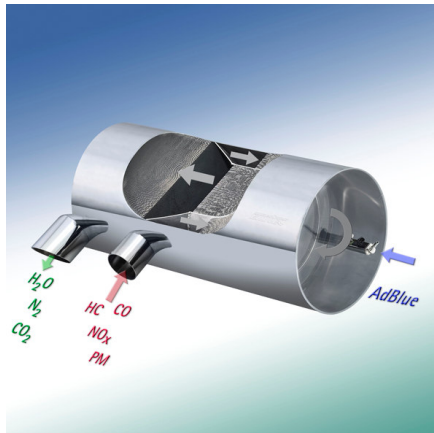
Kompakte SCR-Anlage
